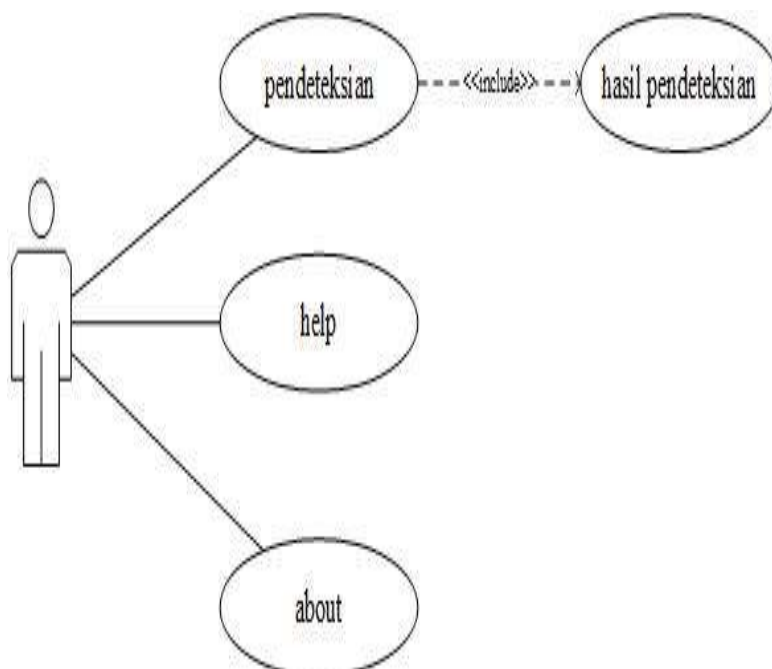
Gambar Use Case Diagram Aplikasi Pendeteksian Madzhab
